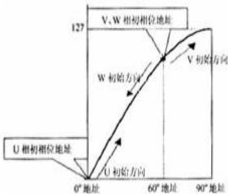
(a) 查正弦函数表原理图
